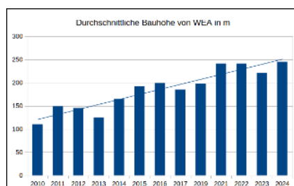
(a) Bauhöhenentwicklung der Windenergieanlagen in A-B-W
