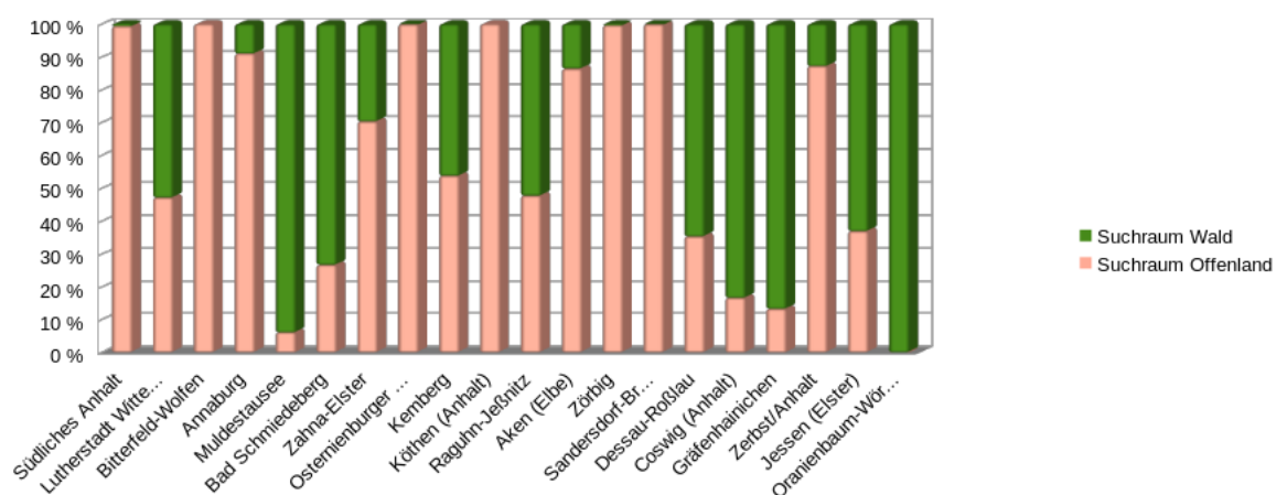
Abbildung 2.7: kommunaler Anteil der Potenzialfläche im Wald
