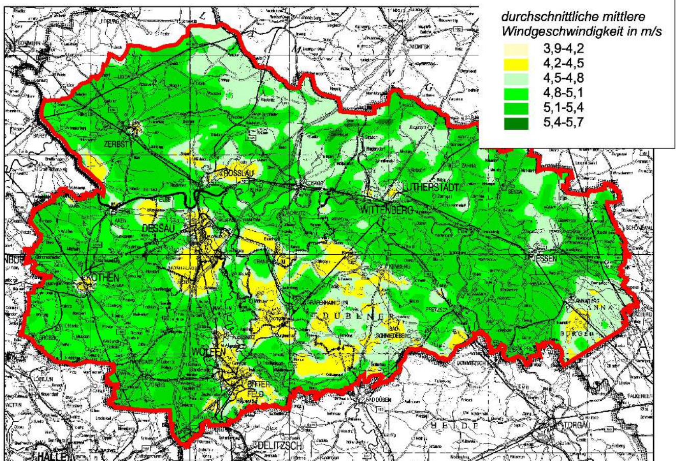
Abbildung 2.3: mittlere Windgeschwindigkeit in der Planungsregion in 80 m über Grund
