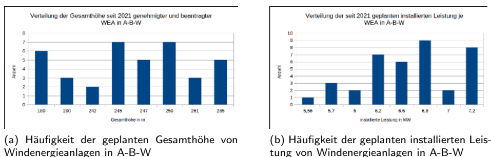
Abbildung 2.1: Häufigkeitsverteilung der Gesamthöhen und Leistungen geplanter Windenergieanlagen in A-B-W
